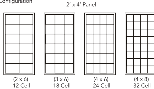
Kwik-Change PLTA/PLNAB Cell Configuration
